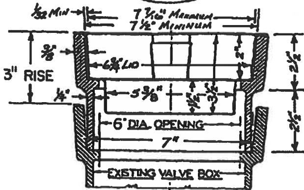
3" PAVADJUSTER
