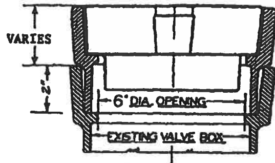
1, 1 1/2, 2, 2 1/2" PAVADJUSTER
